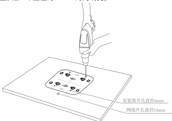
图3-3 钻孔示意图
