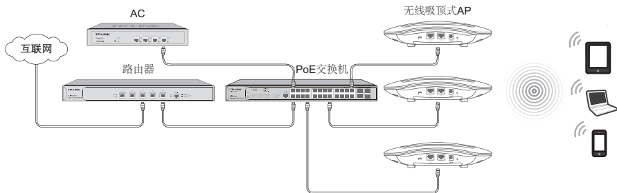
图1-5 典型应用拓扑图-FIT AP模式
