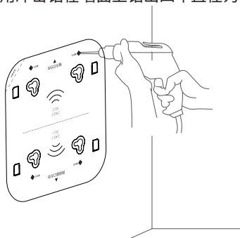
图3-10 钻孔示意图
