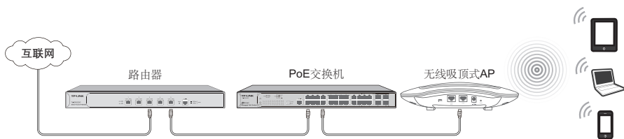
图1-4 典型应用拓扑图-FAT AP模式
