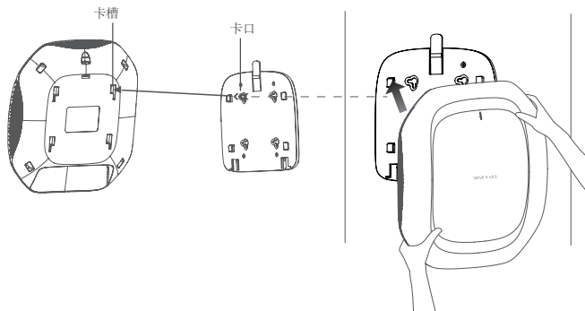
图3-12 安装AP到安装架示意图
