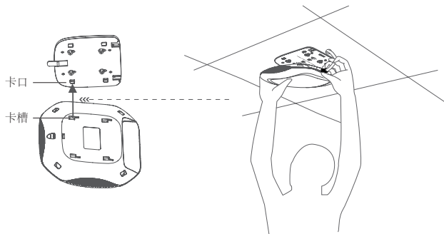
图3-6 安装AP到安装架示意图
