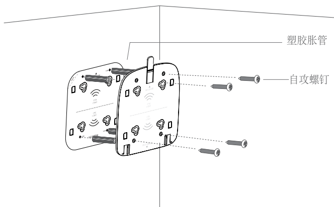
图3-11 固定安装架到墙面示意图
